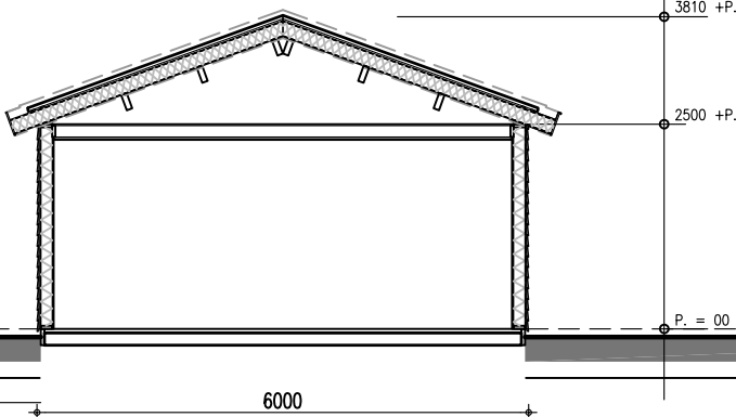
Doorsnede
