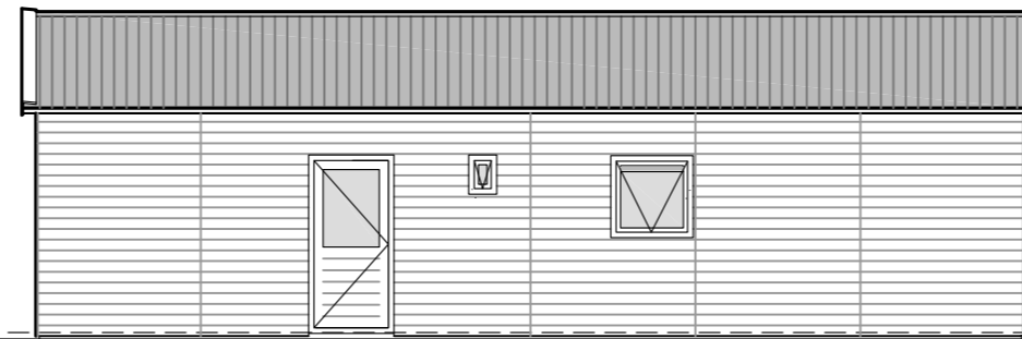
Rechter zijgevel
