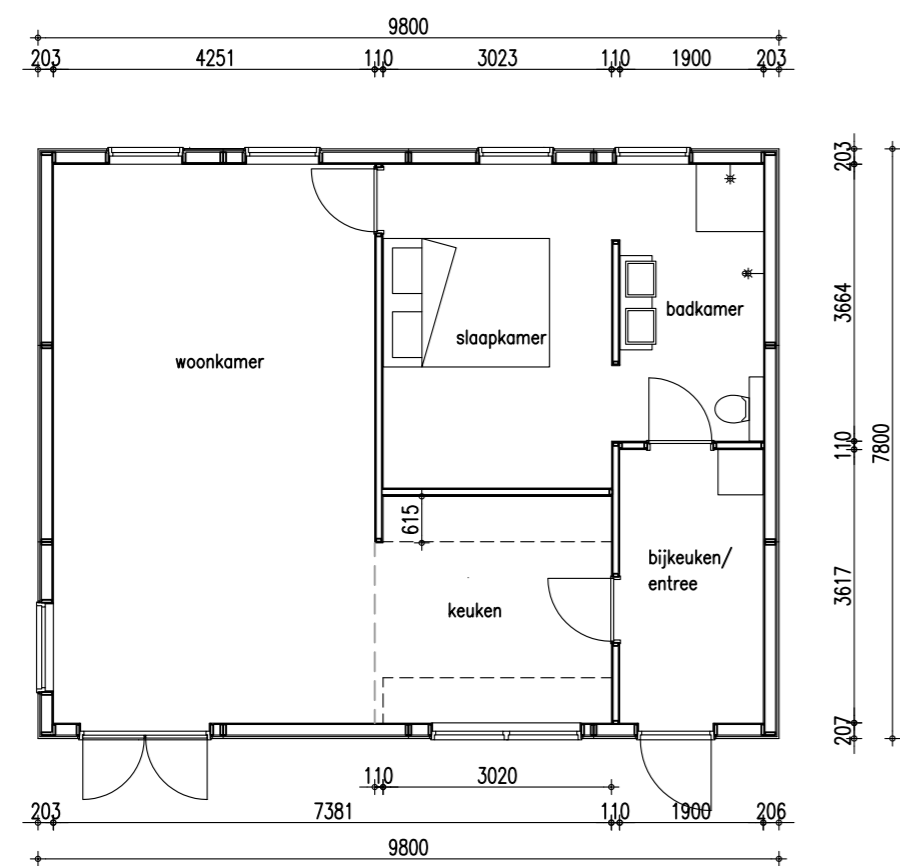
Beganegrond
