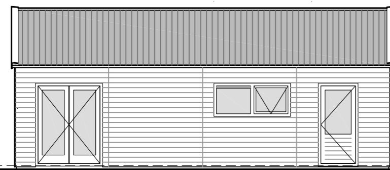
Voorgevel
