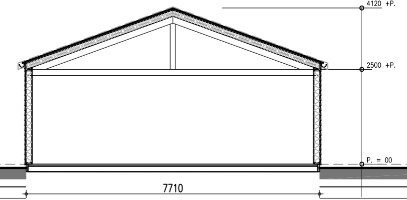
Doorsnede
