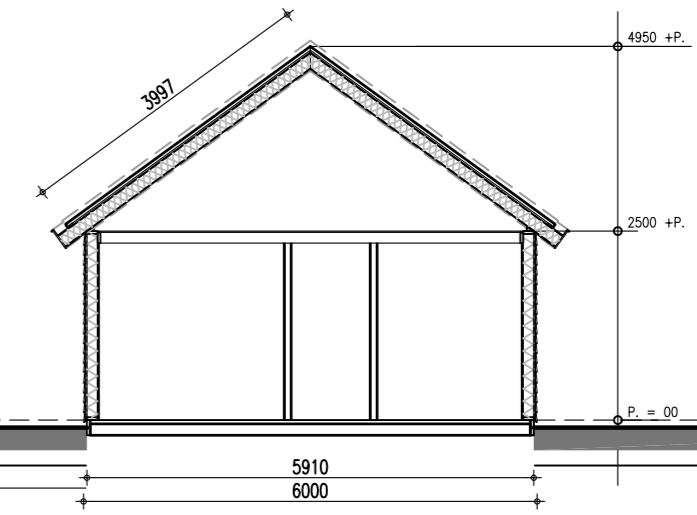
Doorsnede
