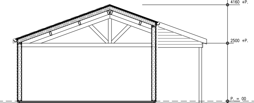
Doorsnede berging
