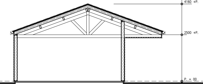
Doorsnede woonkamer
