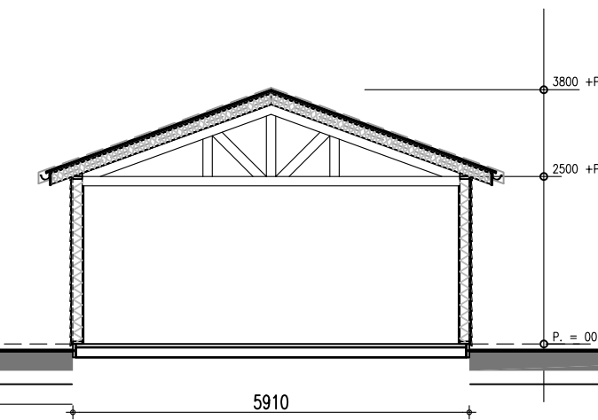
Doorsnede
