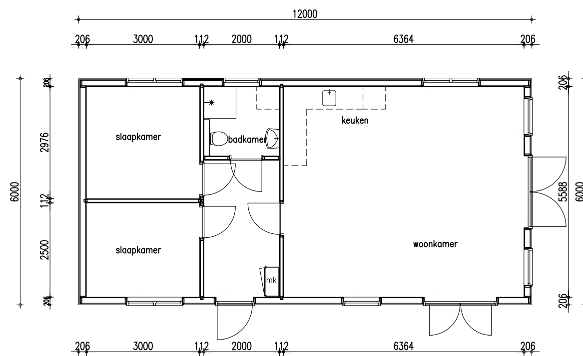
Beganegrond
