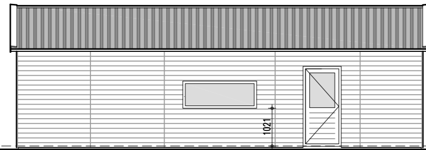
Voorgevel
