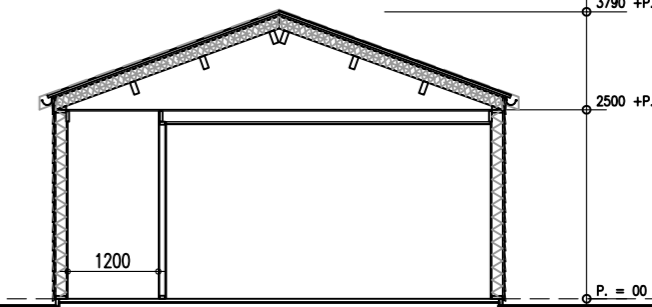
Doorsnede
