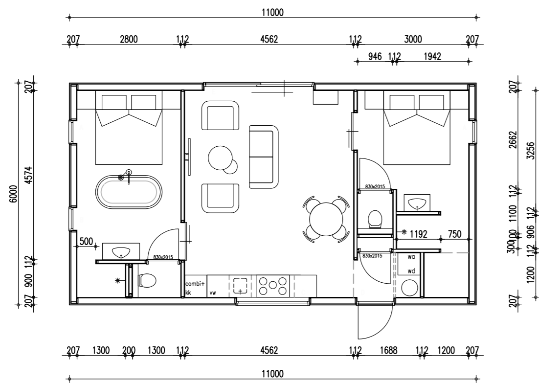
Plattegrond
