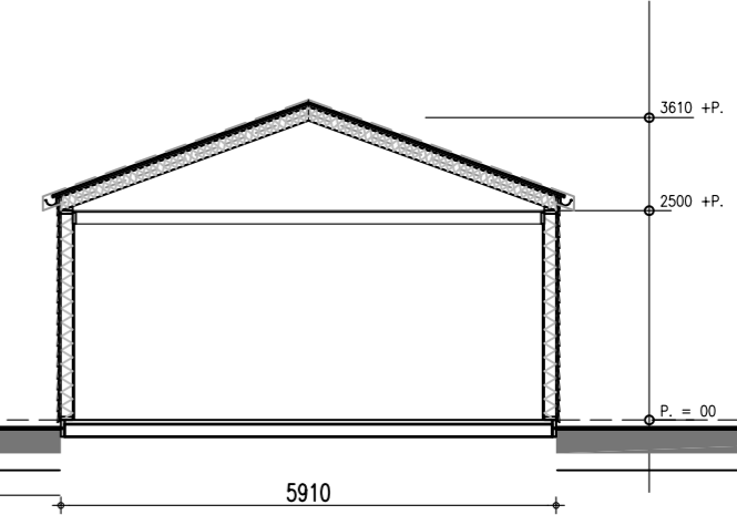
Doorsnede
