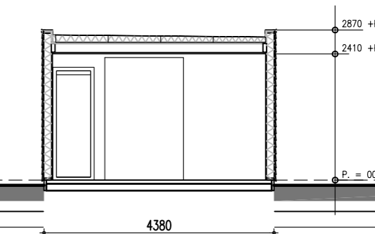
Doorsnede woonkamer
